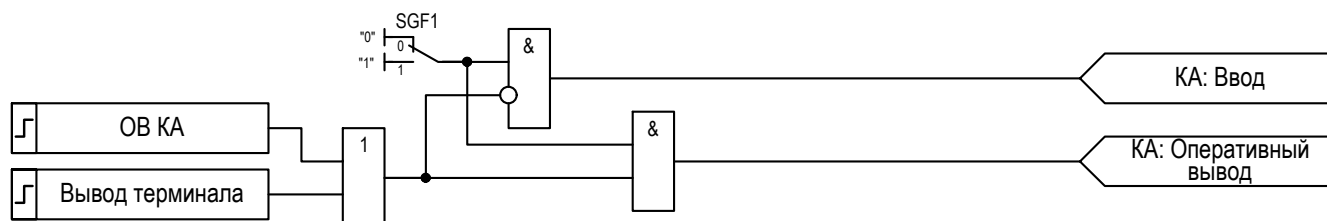
Рисунок 2.26 – Логика управления режимами функционального блока «КА»
